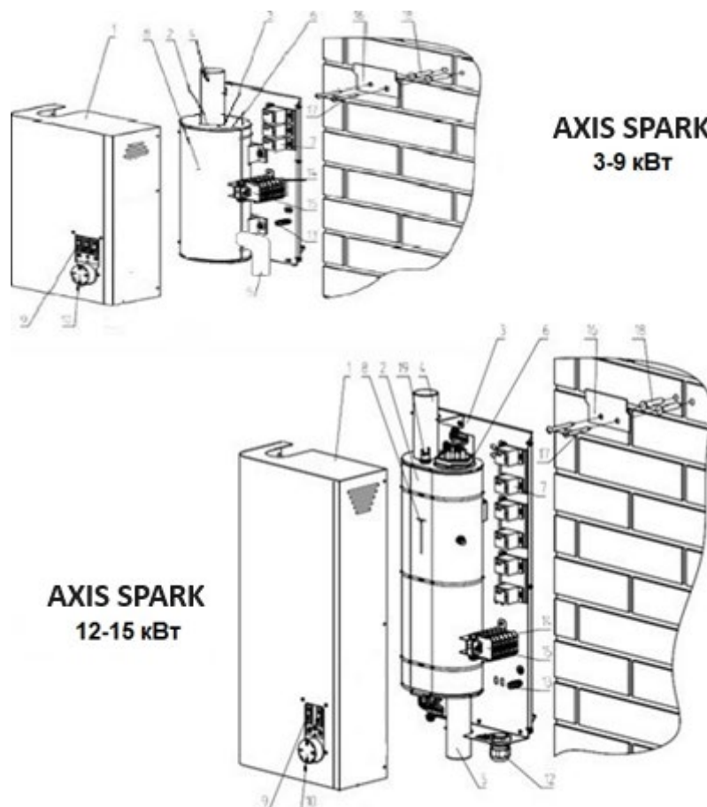
Рис.1 Конструкция котла
