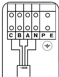
Подключение к трехфазной сети ~380В, 50Гц
