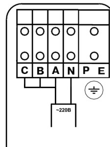
Подключение к однофазной сети ~220В, 50Гц
