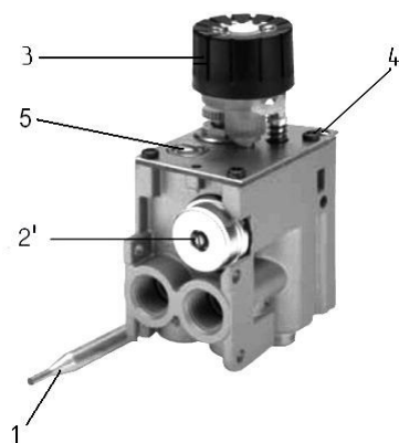
Рисунок 1а - Органы регулировки клапана TGV 307
