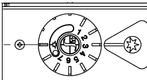
Рисунок 6 – Ручка блока регулятора газовой горелки
