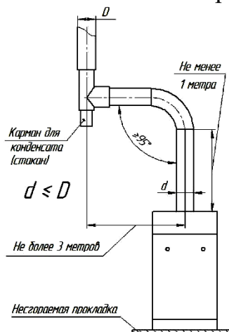
Рисунок 5 – схема монтажа дымохода
