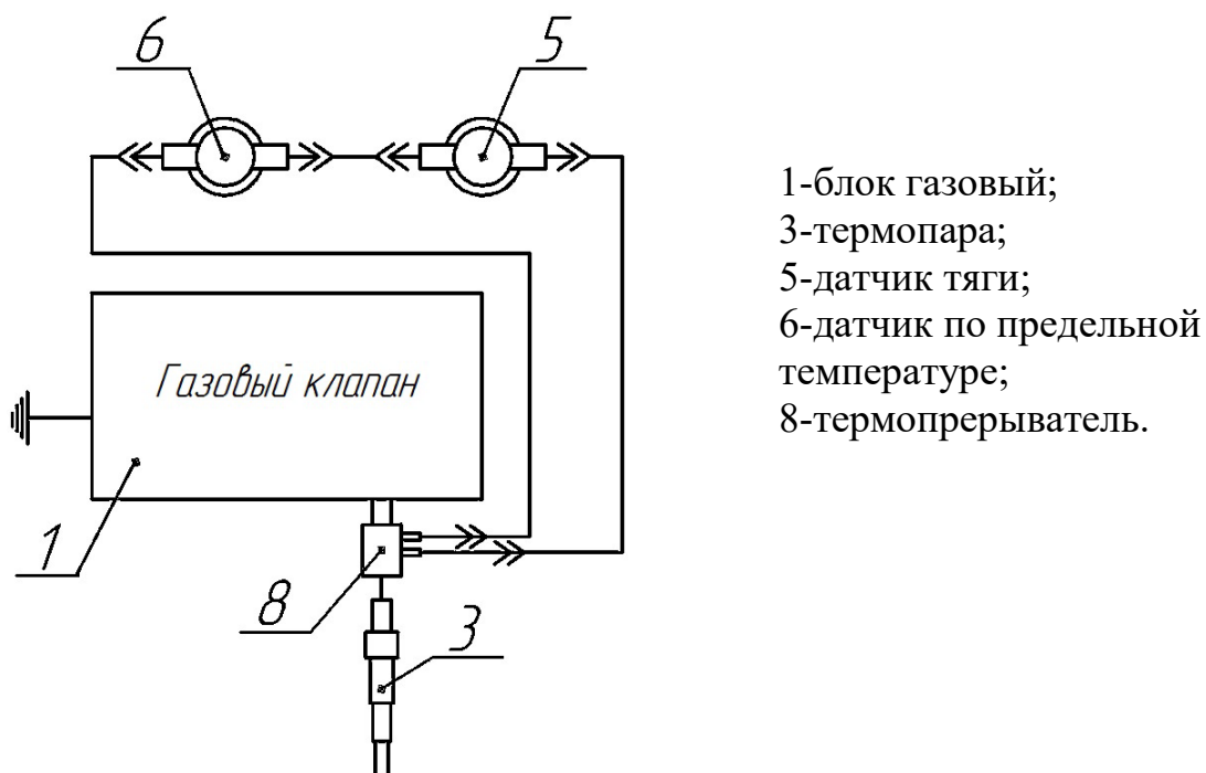
Рисунок 3 – Схема электрическая принципиальная на котел AXIS COMPACT с газовым клапаном
