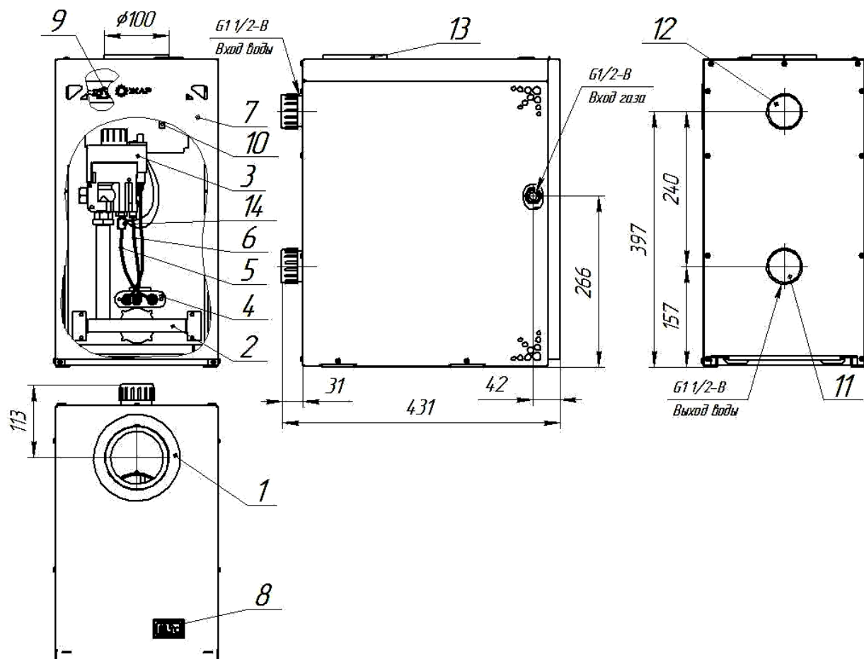
Рисунок 2 – котел AXIS COMPACT
