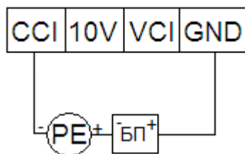
Рисунок 1 схема подключения с внешним источником питания
