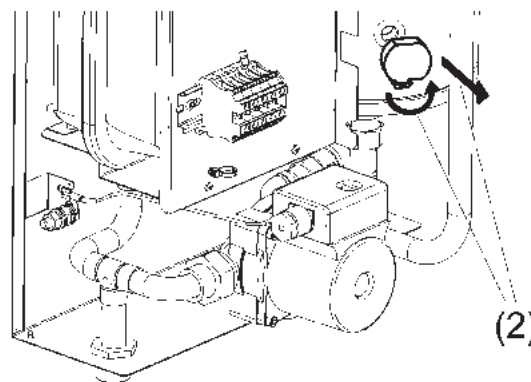
Рисунок 12. Замена датчика давления теплоносителя
