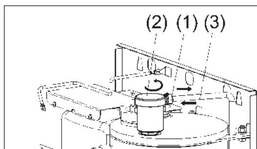
Рисунок 15. Замена автоматического воздухоотводчика
