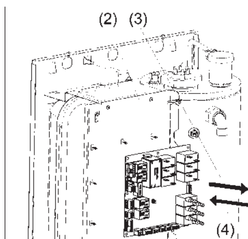
Рисунок 17. Замена платы контроллера
