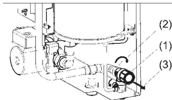
Рисунок 14. Замена предохранительного клапана
