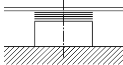
Fig. 6: Компенсационные шайбы на поверхности фундамента
