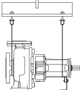
Fig. 3: Строповка насоса
