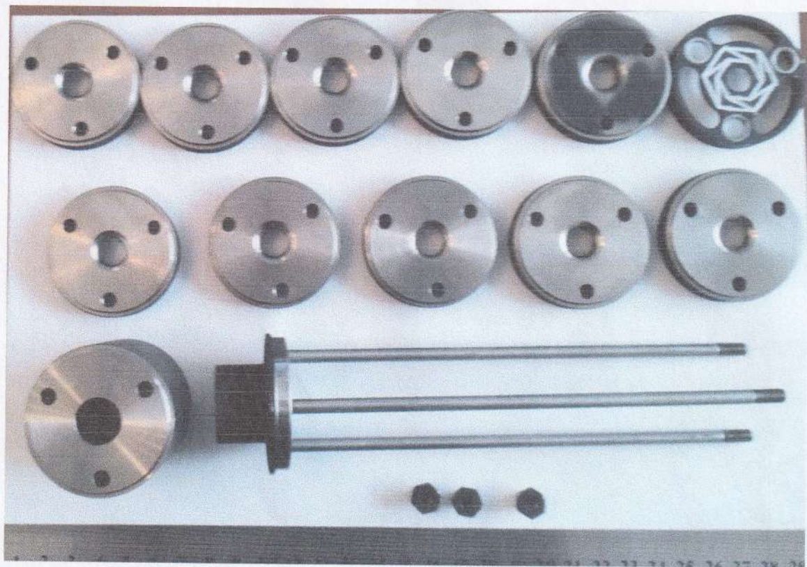
Фото №4. Представленный на исследование объект («пламегаситель Гексагон») после разборки.
