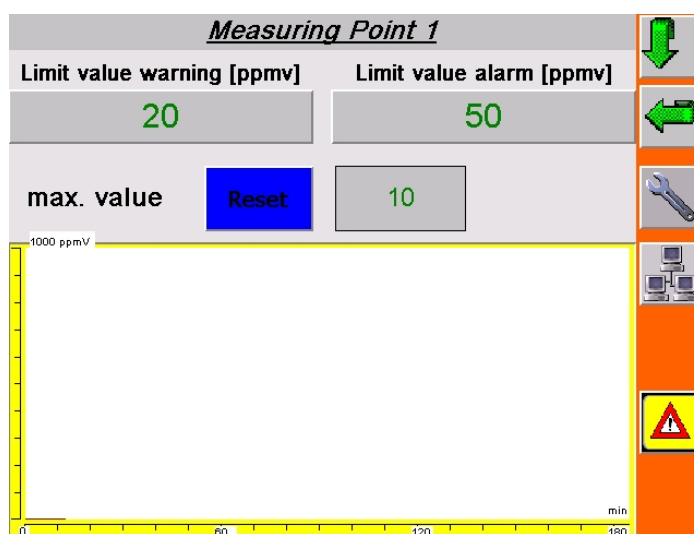
Рис. 5.3 меню точки измерения 1
