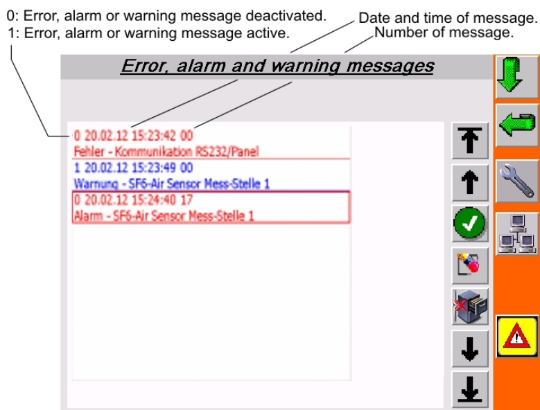
Рис. 5.4 Сообщения об ошибках, тревоге и предупреждения.
