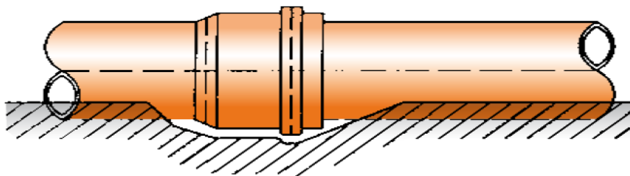
Рис. 4 Углубление под раструбом
