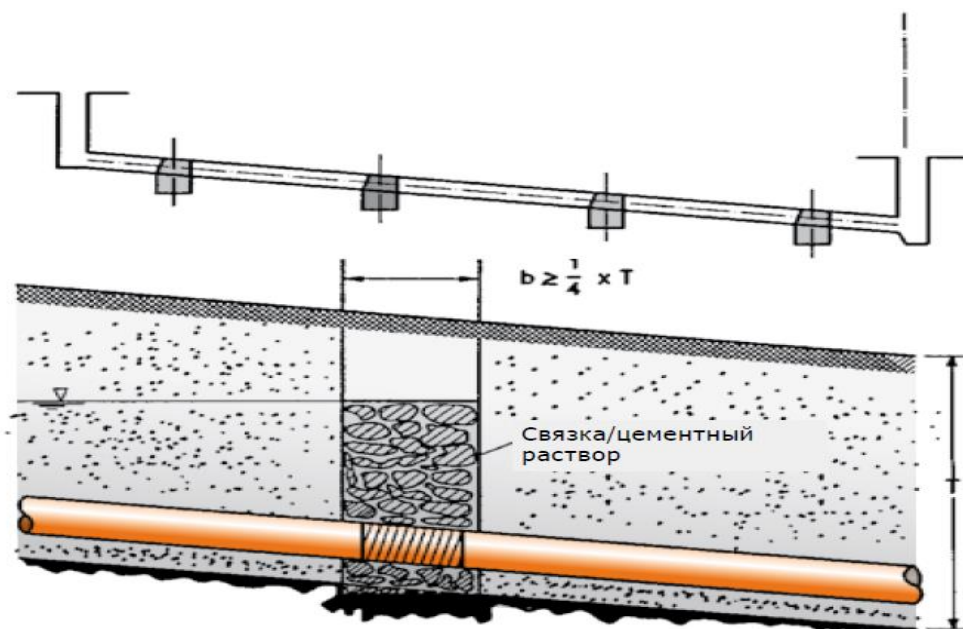
Рис. 8 Прокладка труб в крутых склонах
