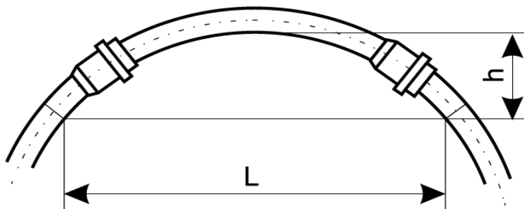
Рис. 2 Изогнутый трубопровод
