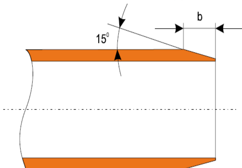
Рис. 1 Скос вставляемого конца трубы
