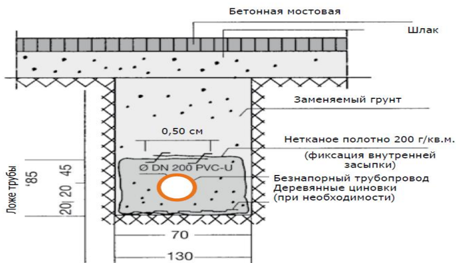
Рис. 7 Пример прокладки труб в мягком грунте
