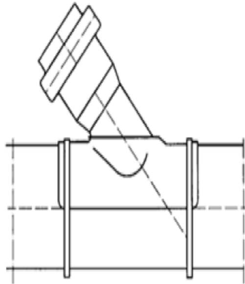
Рис. 15 Приклеиваемая накладка с раструбом
