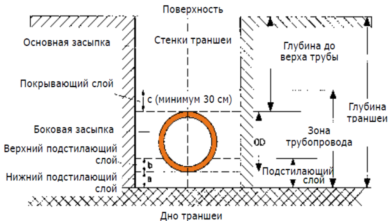
Рис. 3 Устройство траншеи
