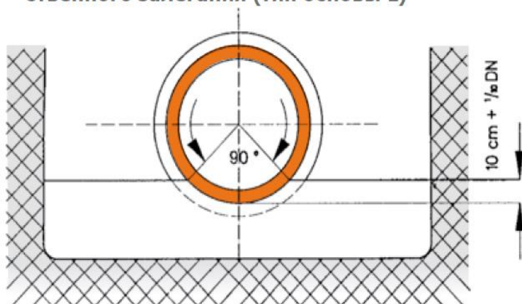
Рис. 6 Укладка в ненарушенный грунт естественного залегания (тип основы 1)
