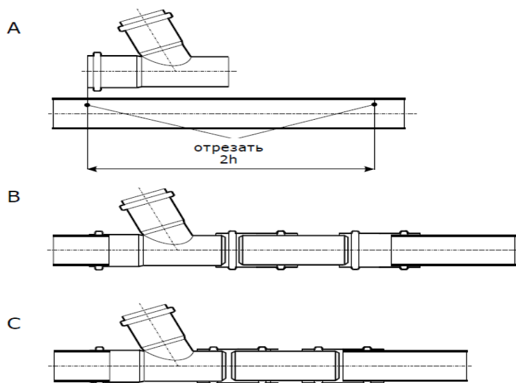
Рис. 14 Установка дополнительного тройника
