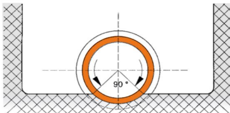
Рис. 5 Укладка в ненарушенный грунт естественного залегания (тип основы 2)
