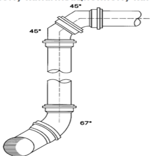
Рис. 12 Пример вертикального подключения к главному канализационному каналу
