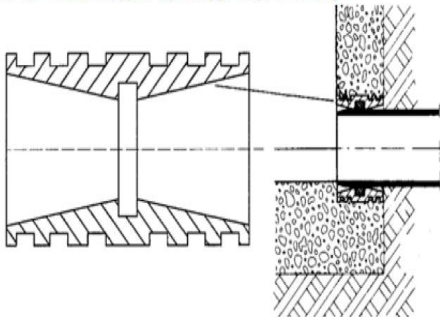
Рис. 13 Гильза для прохода через стену
