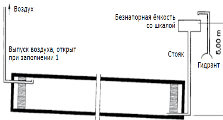
Рис. 10 Проверка герметичности
