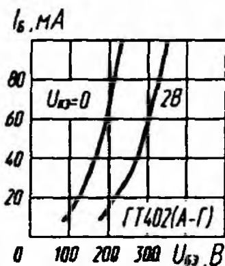
Входные характеристики
