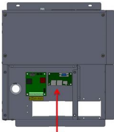
Параллельная плата
