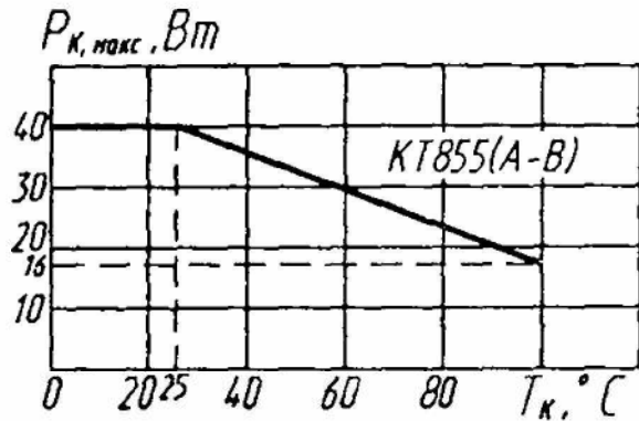
Зависимость максимально допустимой постоянной рассеиваемой мощности коллектора от температуры корпуса
