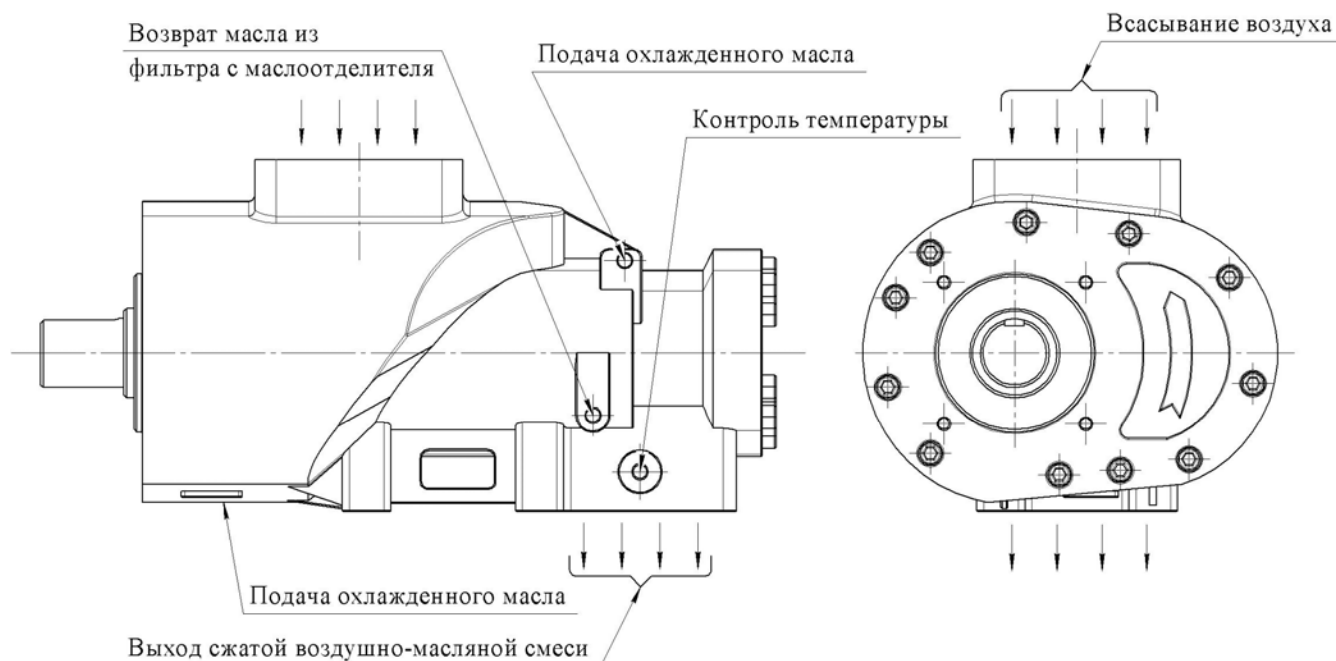
Общий вид винтового блока CF90LD1:
