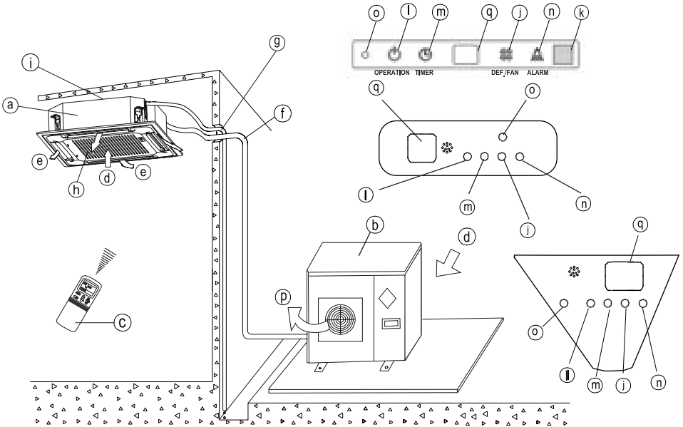
Панель управления и индикации внутреннего блока
