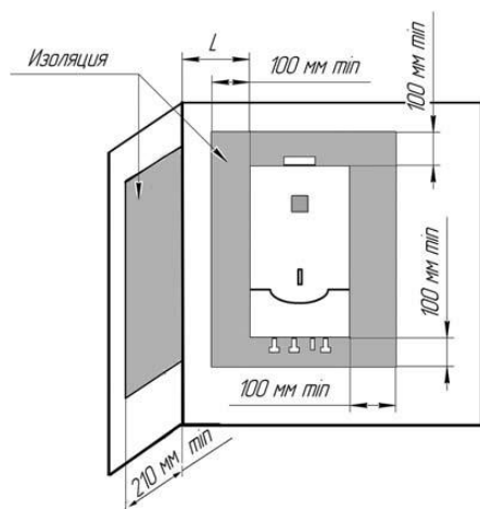
Рис. 5 Установка аппарата на трудносгораемых стенах.
