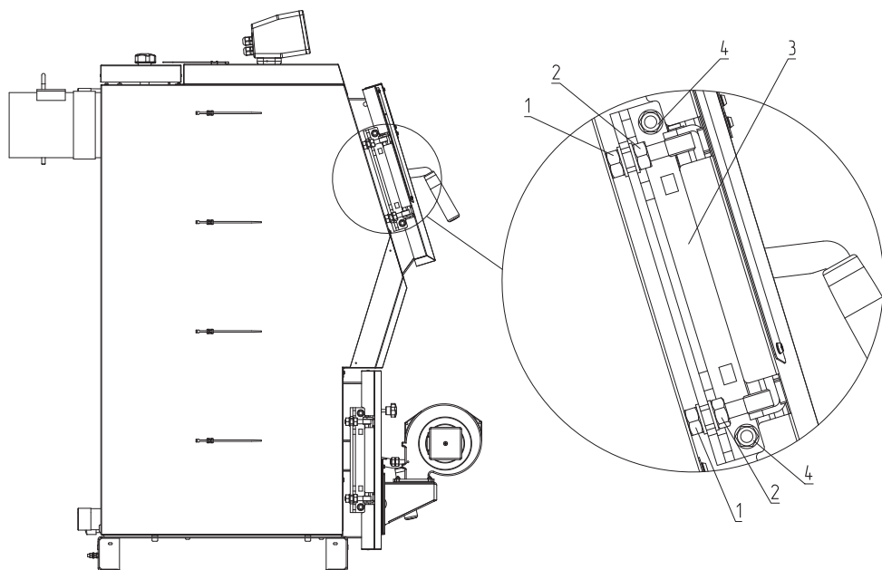
Рис.14 Регулировки петли дверцы загрузочной
