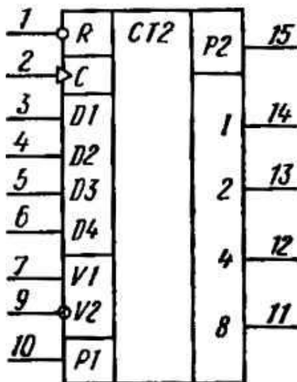
Условное графическое обозначение К555ИЕ18
