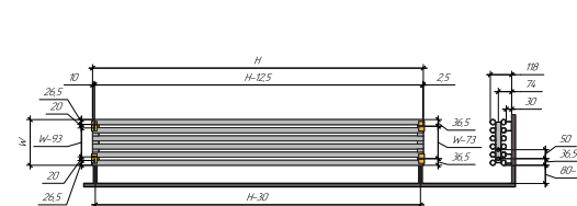
Горизонтальная напольная
