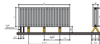
Вертикальная напольная
