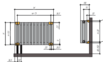
Вертикальная напольная
