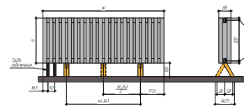
Вертикальная напольная
