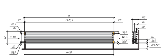
Горизонтальная напольная
