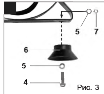
4 – болт 6 – присоска 5 – шайба 7 – гайка.
