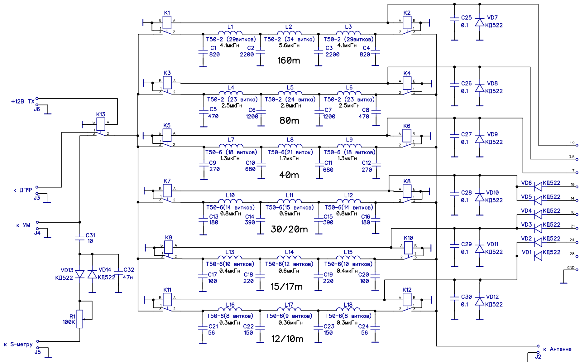
Фильтры нижних частот трансивера ФНЧ-3М
