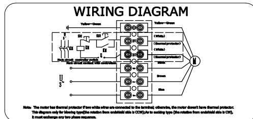
WIRING DIAGRAM (接线图) :
