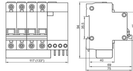
Рисунок В.2 – Габаритные, установочные и присоединительные размеры четырехполюсного АВДТ типа АД14
