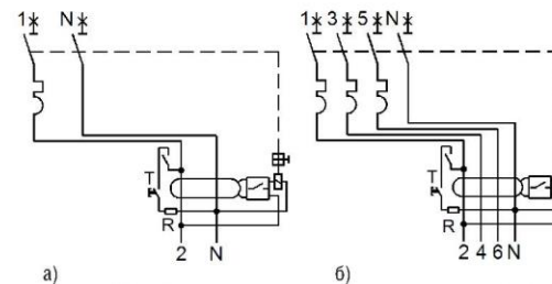
а) Рисунок Г.1 – Принципиальные электрические схемы АВДТ а) двухполюсного; б) четырехполюсного Т – устройство эксплуатационного контроля (кнопка «ТЕСТ») R – токоограничивающее сопротивление
