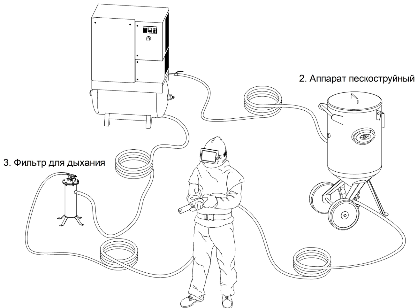
Рисунок 1 – Схема подключения
