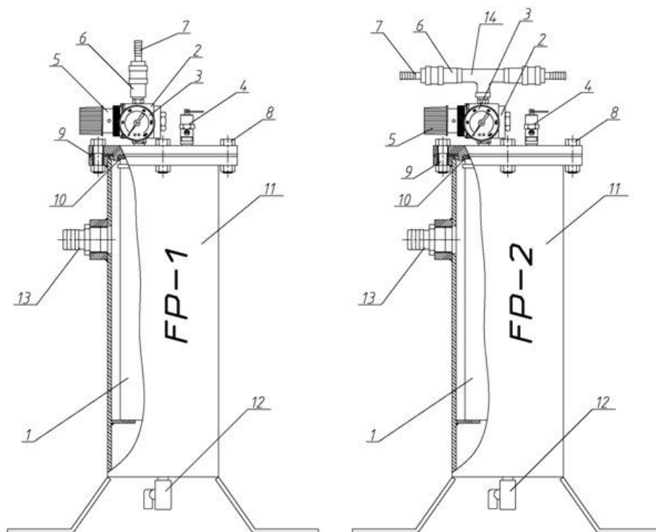
Рисунок 2 - Фильтр воздушный патронный «FP»
