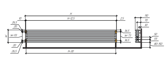
Горизонтальная напольная
