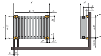
Вертикальная напольная
