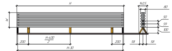
Горизонтальная напольная
