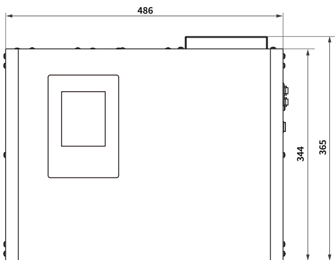
Рубин ТСН-12000
