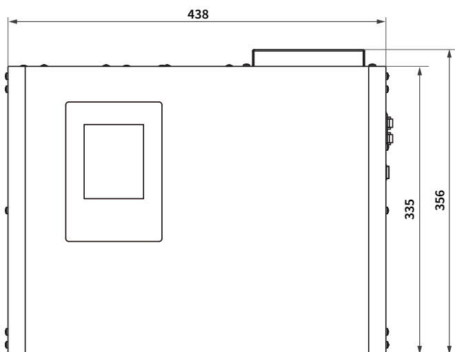
Рубин ТСН-5000
