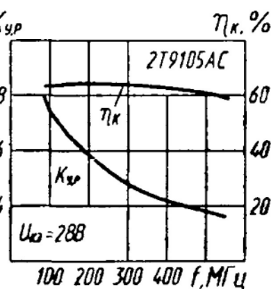
Зависимости коэффициента усиления и коэффициента полезного действия от частоты
