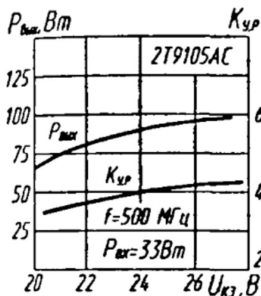
Зависимости выходной мощности и коэффициента усиления от напряжения коллектор—эмиттер
