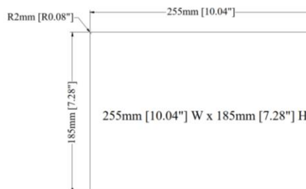
Cutout Dimensions
