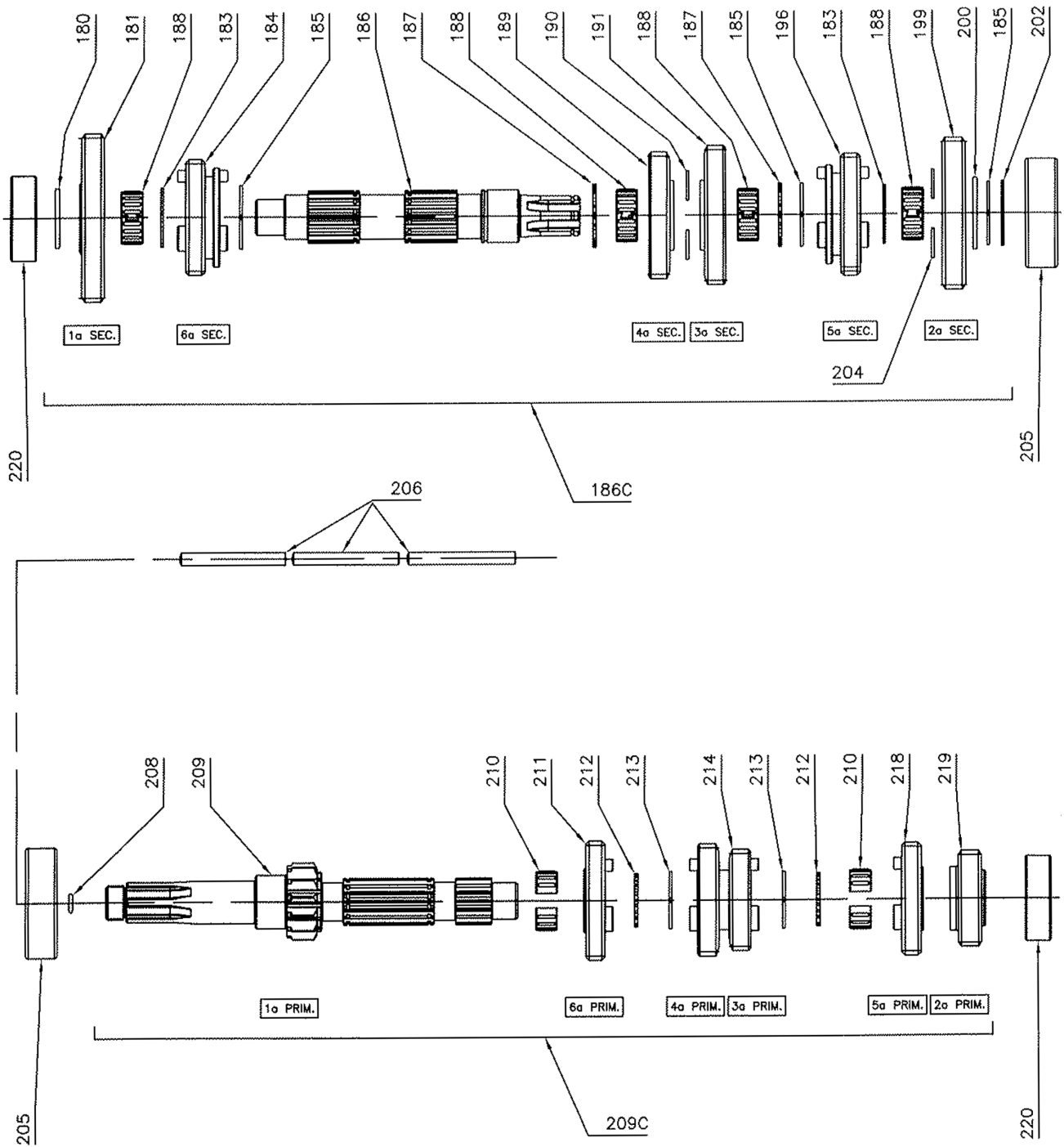
222 ALBERI PRIMARIO E SECONDARIO COMPLETI CON CUSCINETTI PRIMARY AND SECONDARY SHAFTS COMPLETE WITH BEARINGS ARBRES PRIMAIRE ET SECONDAIRE COMPLETS AVEC ROULEMENTS
