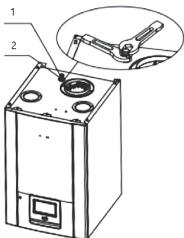
Рис. 3 Демонтаж заглушки.
