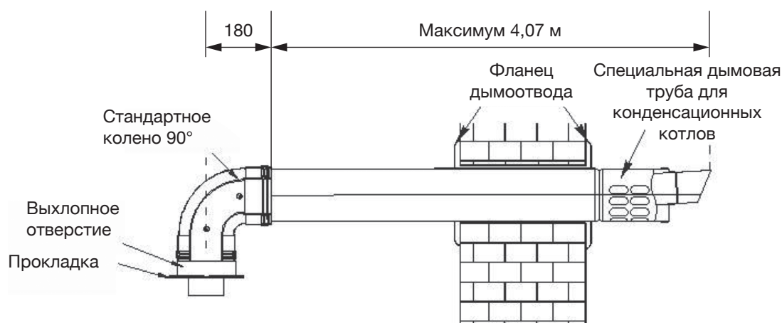
Рис. 40. Пример монтажа схемы C13.
