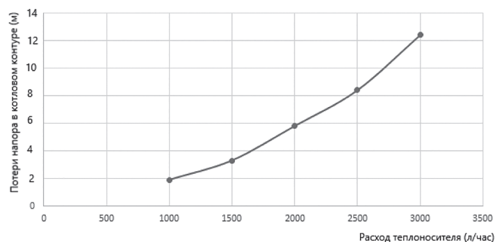
Рис. 42. Потери давления в котловом контуре.
