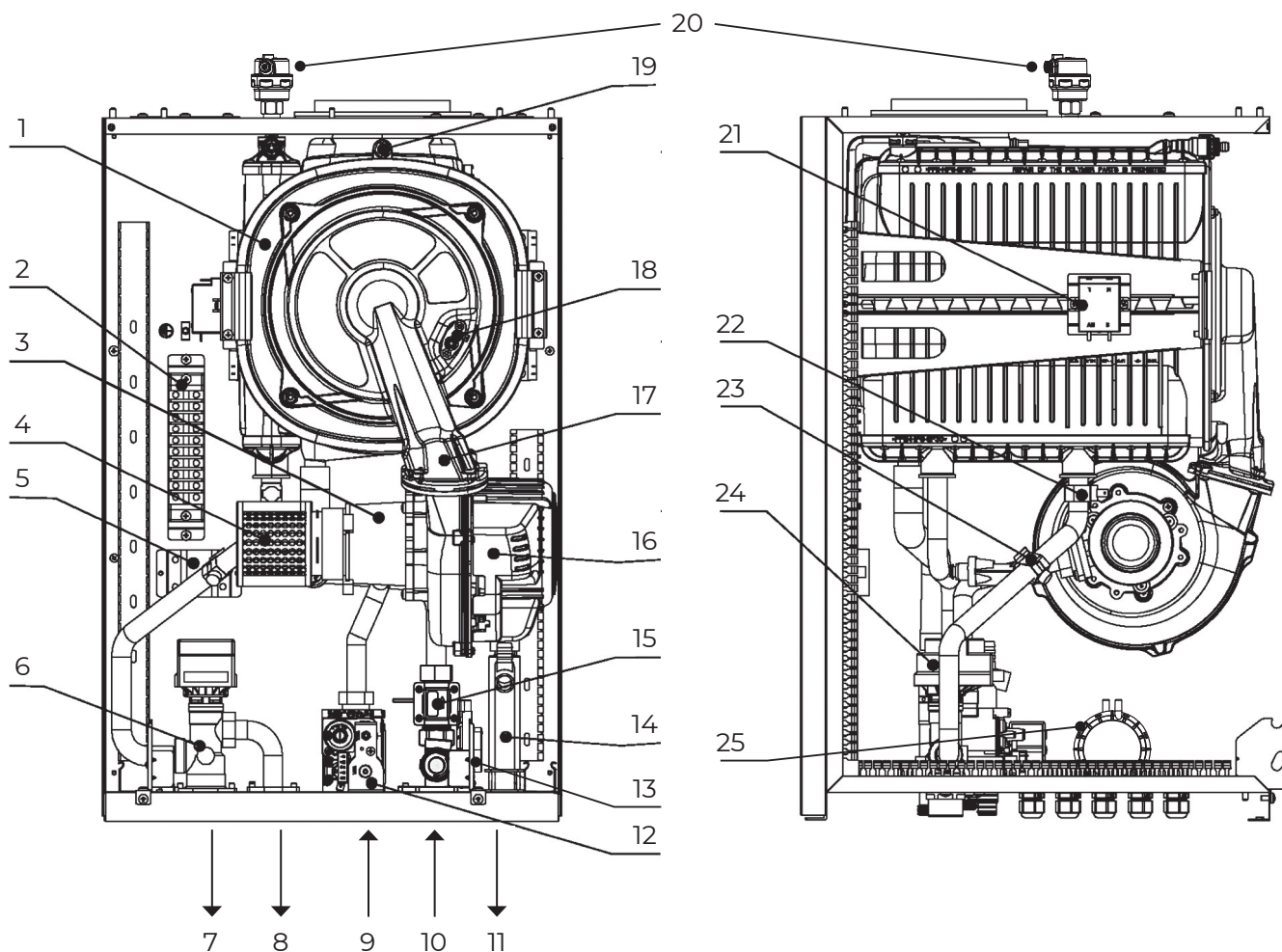
Рис. 2. Общая схема.
