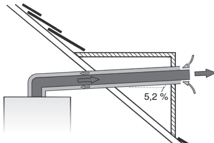
Рис. 39. Угол наклона дымохода.
