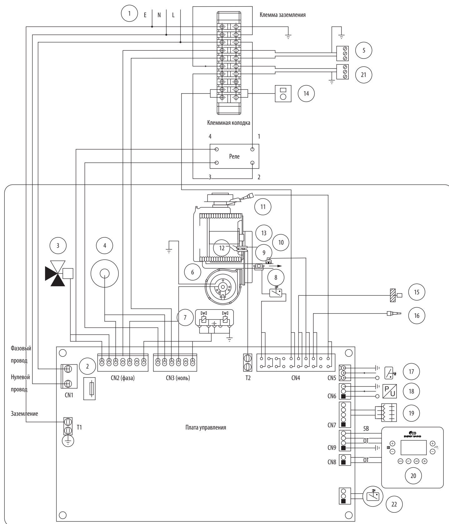
Рис. 41. Электрическая схема платы.
