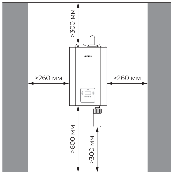
Рис. 38. Рекомендуемые расстояния для монтажа
