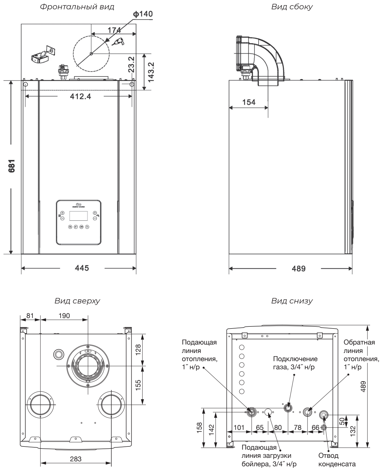
Рис. 37. Монтажные размеры.
