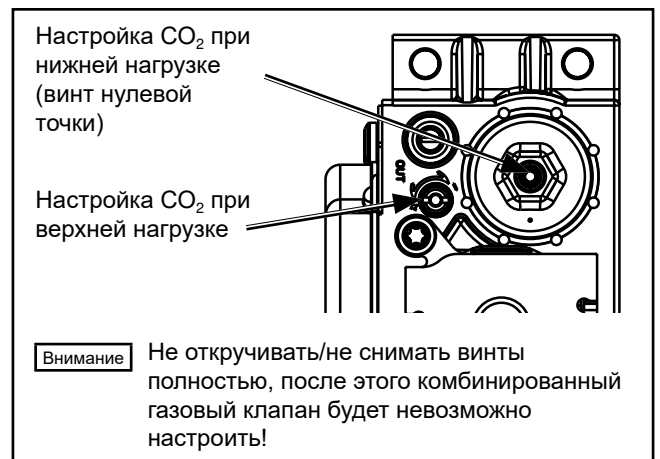
Рисунок: Комбинированный газовый клапан
